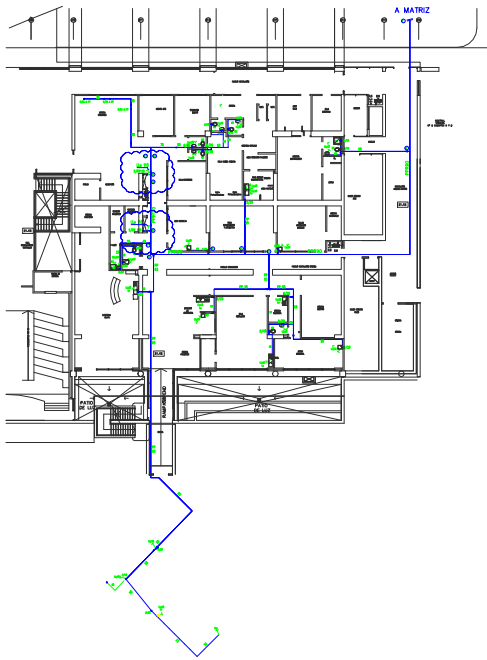
AGUA FRÍA
